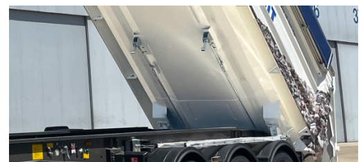
Sistema rápido para abertura dos fechos de porta
